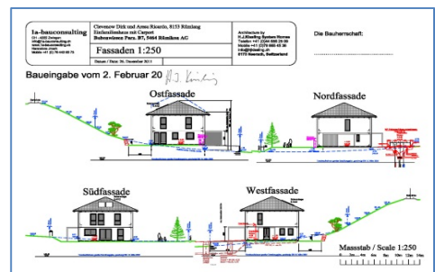
Fassadenplan Fertighaus
